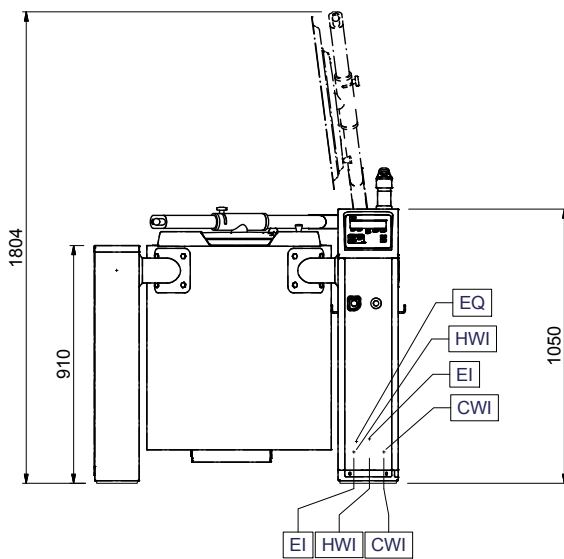
Zij aanzicht
